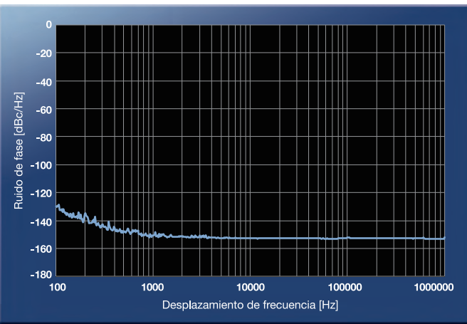
Ruido de fase TX (banda de 14 MHz, Modo: CW)
