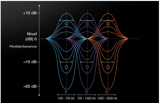
Ilustración conceptual del ecualizador paramétrico de 3 etapas
